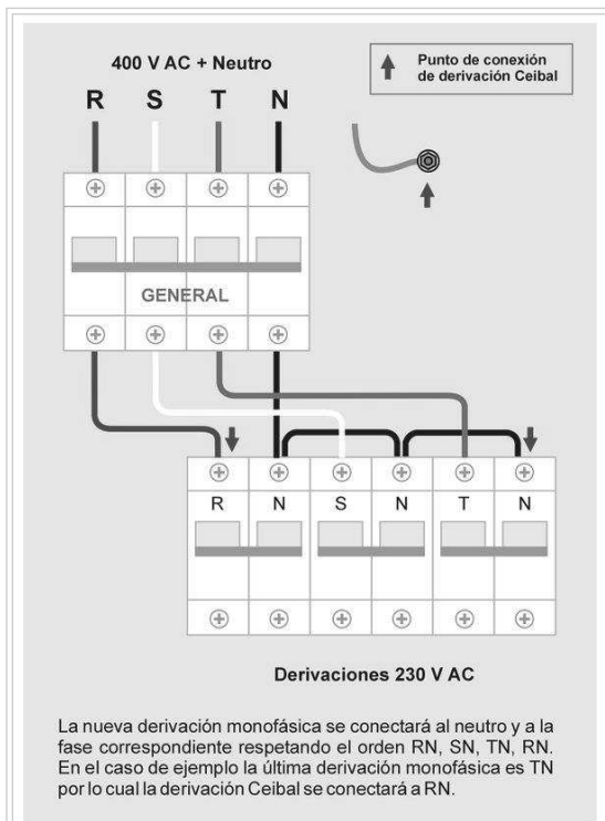
Fig. 4 - Puntos de conexión de derivación monofásica 230 V AC en tablero con suministro tetrapolar 400 V AC + Neutro
