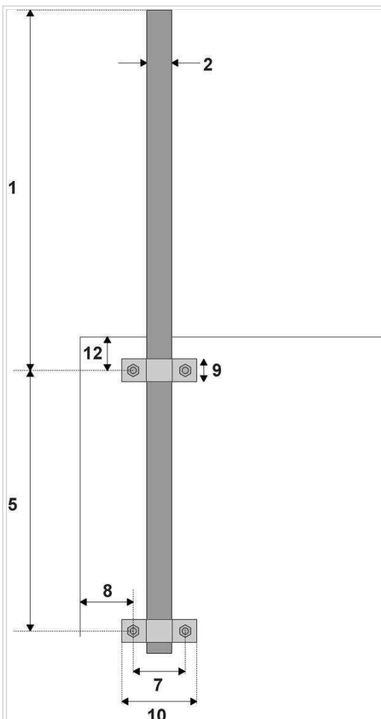
Fig. 2 : Principales dimensiones
