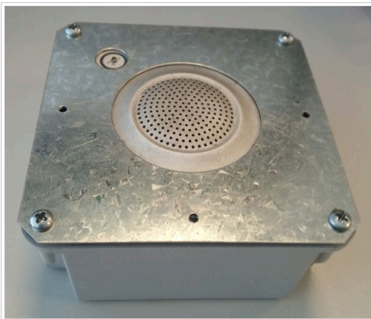
Fig. 19 : Micrófono en caja con tapa de chapa.
