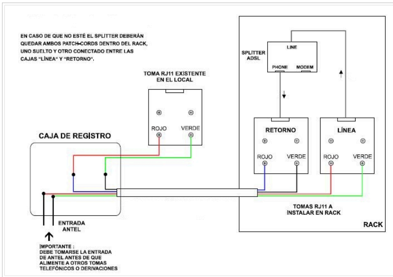
Fig. 2 - Diagrama de instalación telefónica (no vigente)
