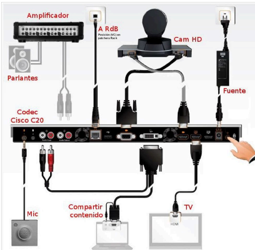
Fig. 21 : Interconexión de equipos con Codec Cisco C20.
