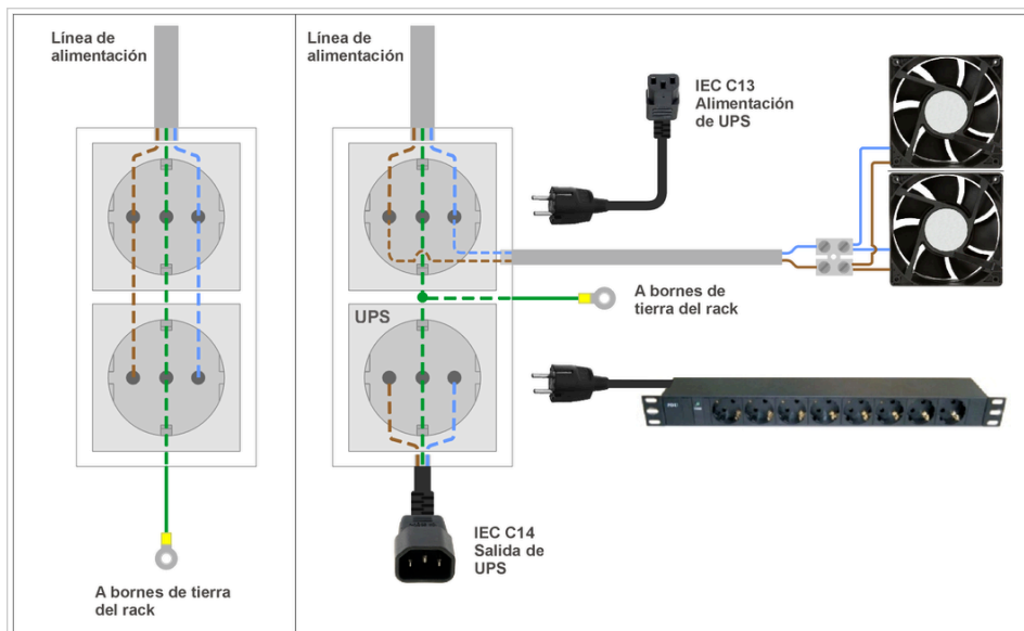
Fig. 3 : Diagrama de instalación eléctrica del rack
