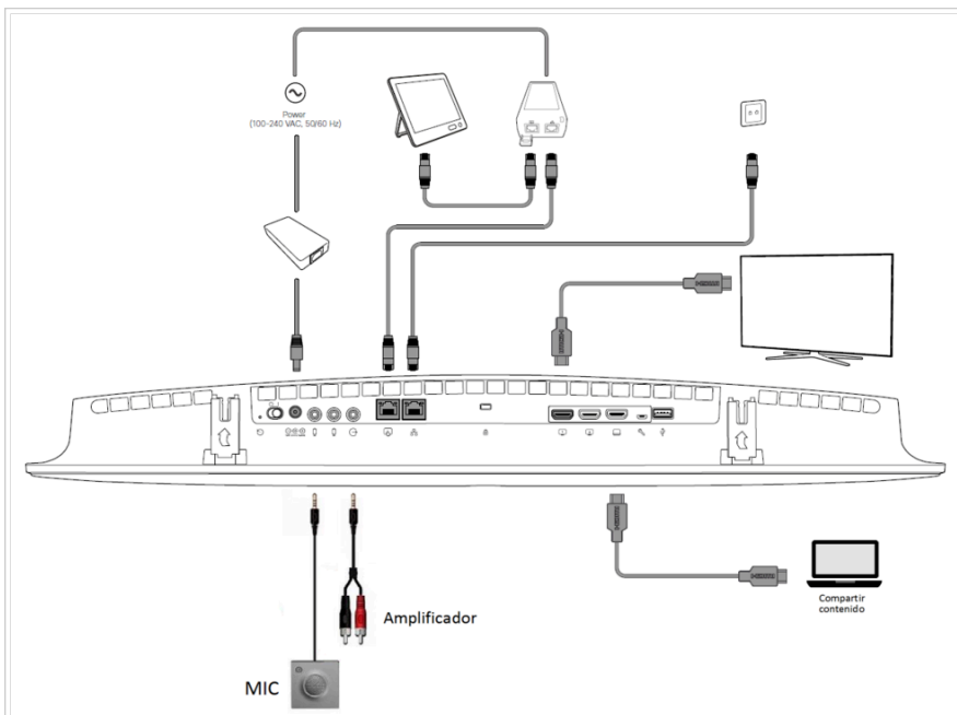
Fig. 23 : Interconexión de equipos con Roomkit Cisco -adaptado de guía de instalación Cisco-.
