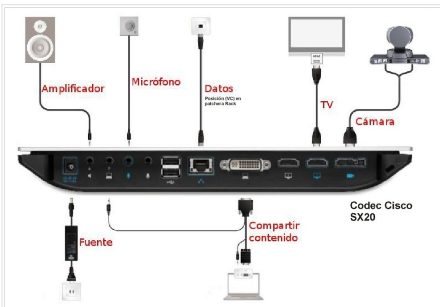
Fig. 22 : Interconexión de equipos con Codec Cisco SX20.
