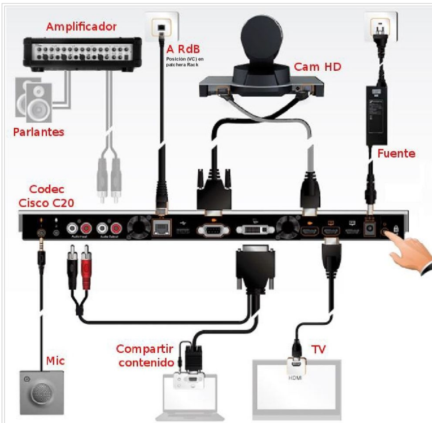
Fig. 21 : Interconexión de equipos con Codec Cisco C20.
