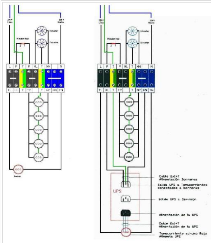
Fig. 5 : Diagrama eléctrico de bandeja con bornera
