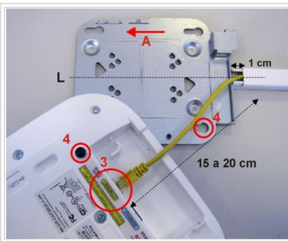
Fig. 4 - Conexión de AP
