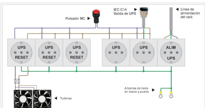
Fig. 7 : Diagrama eléctrico de bandeja sin bornera
